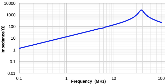
CSEB0420H-2R2M
