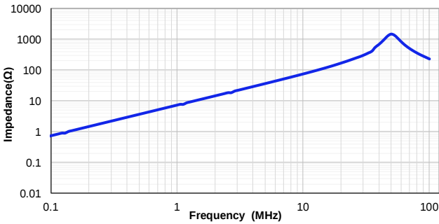
CSEB0420H-1R2M
